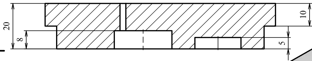
A-A (1:1)
