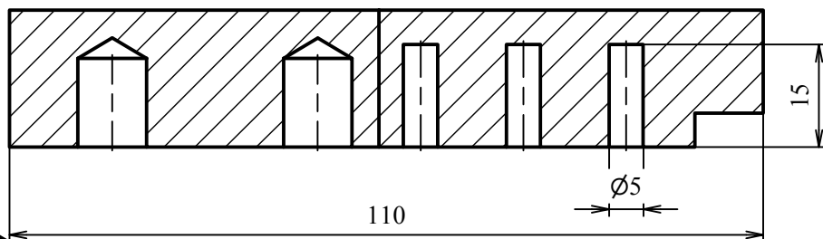
T-T (1 : 1)
