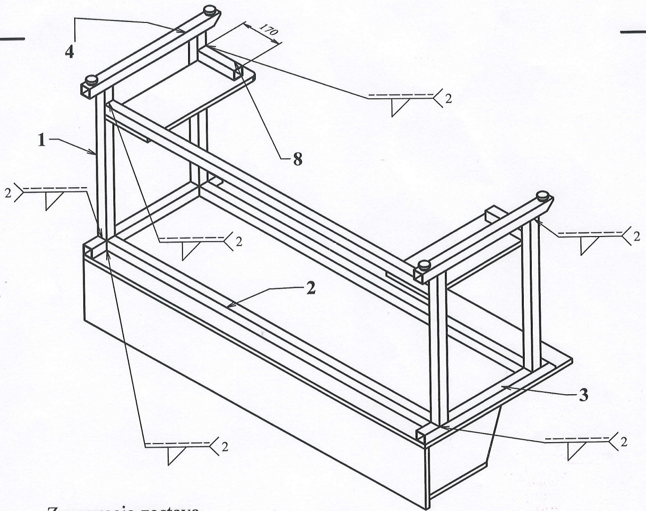
Zvarovacia zostava
